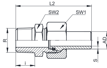
焊接式接头
