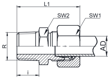
卡套式接头
