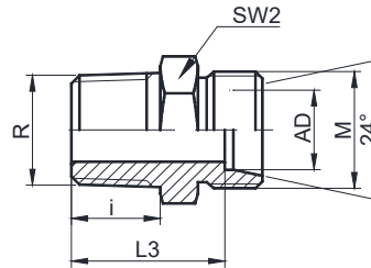
接头体
