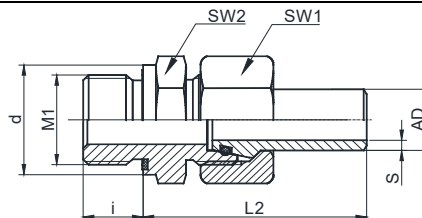
焊接式接头
