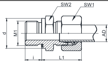
卡套式接头
