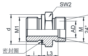
接头体
